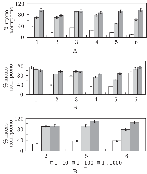
Рис. 3. Вплив водних витяжок різної концентрації з листків (А), стебел (Б) та коренів (С) на ріст коренів амаранту: 1 — Alnus subcordata ; 2 — A. subcordata (дворічні рослини); 3 — A. barbata ; 4 — A. incana f. pinnatifida ; 5 — A. incana f. pendula (дворічні рослини); 6 — A. glutinosa (дворічні рослини)
